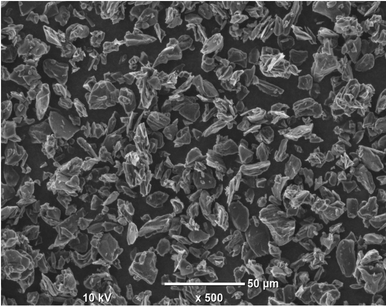
产品电镜图(Product SEM)
