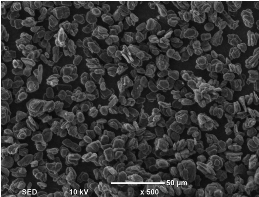
产品电镜图(Product SEM)
