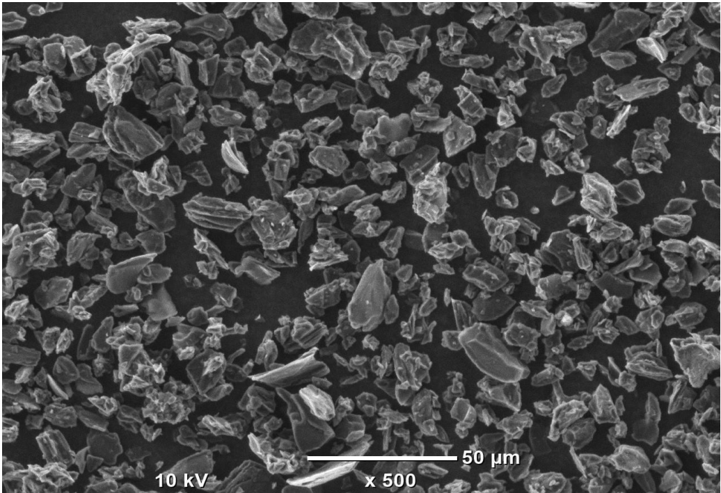
产品电镜图(Product SEM)
