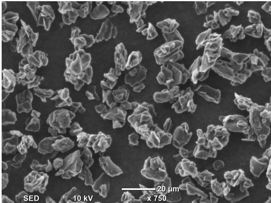
LT-ZH-9X 人造石墨电镜图(SEM)
