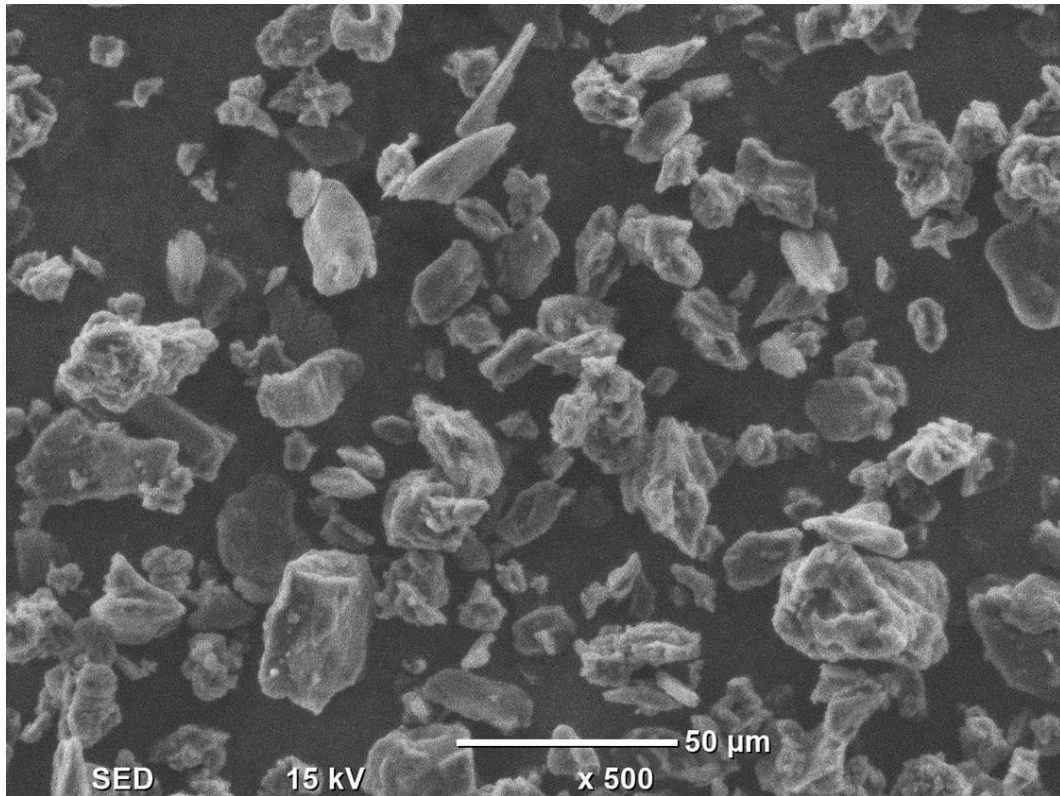
LT-ZH-916 人造石墨电镜图(SEM)
