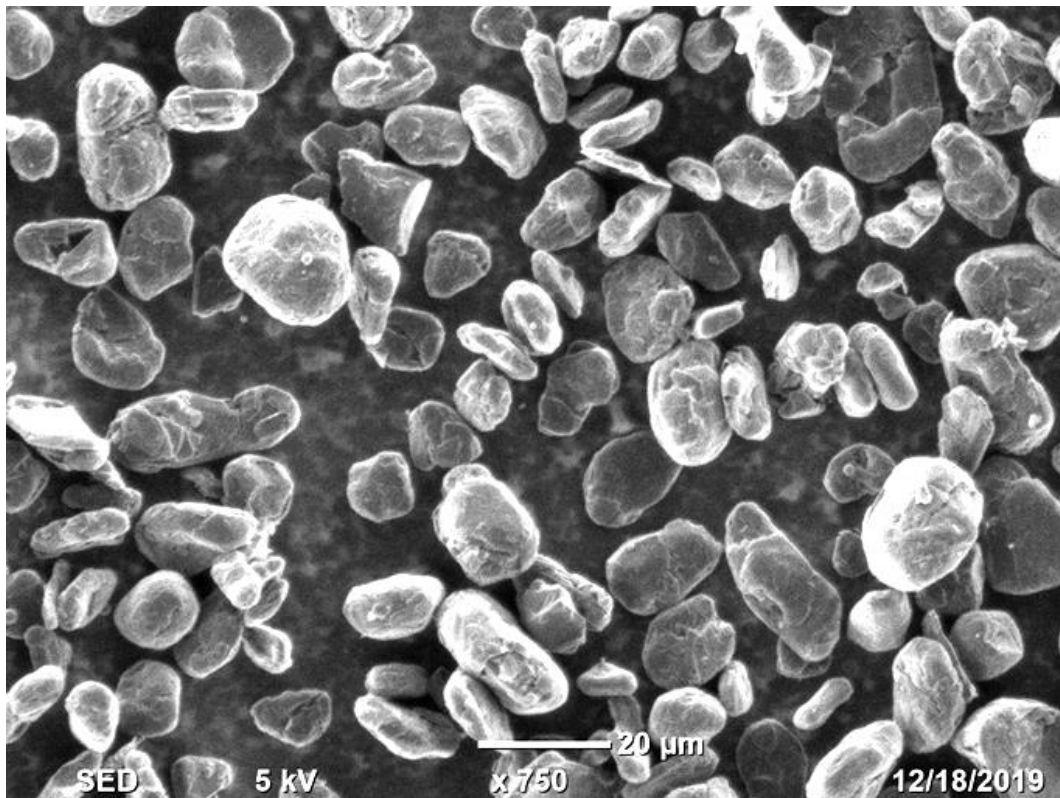
LT-N98 天然石墨电镜图(SEM)
