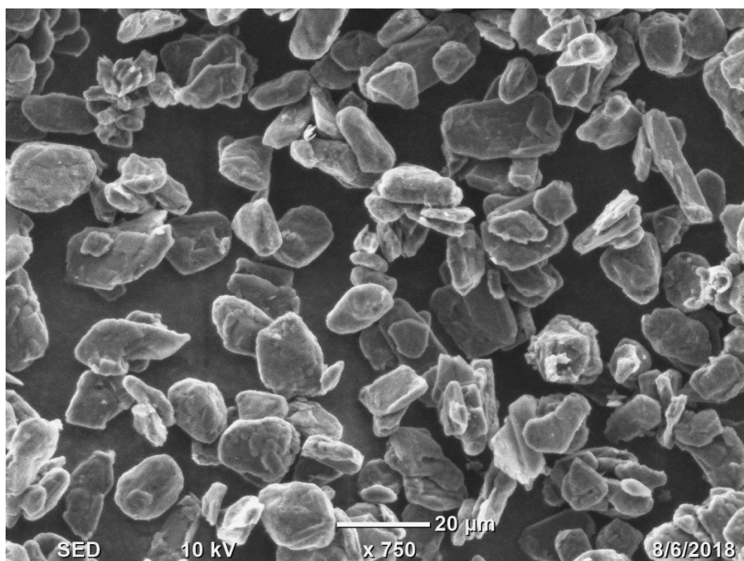
LT-N8 天然石墨电镜图(SEM)
