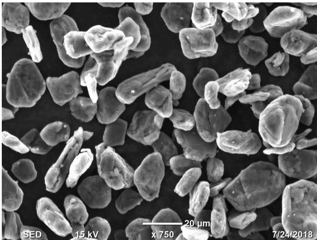
LT-N58-30C 天然石墨电镜图(SEM)
