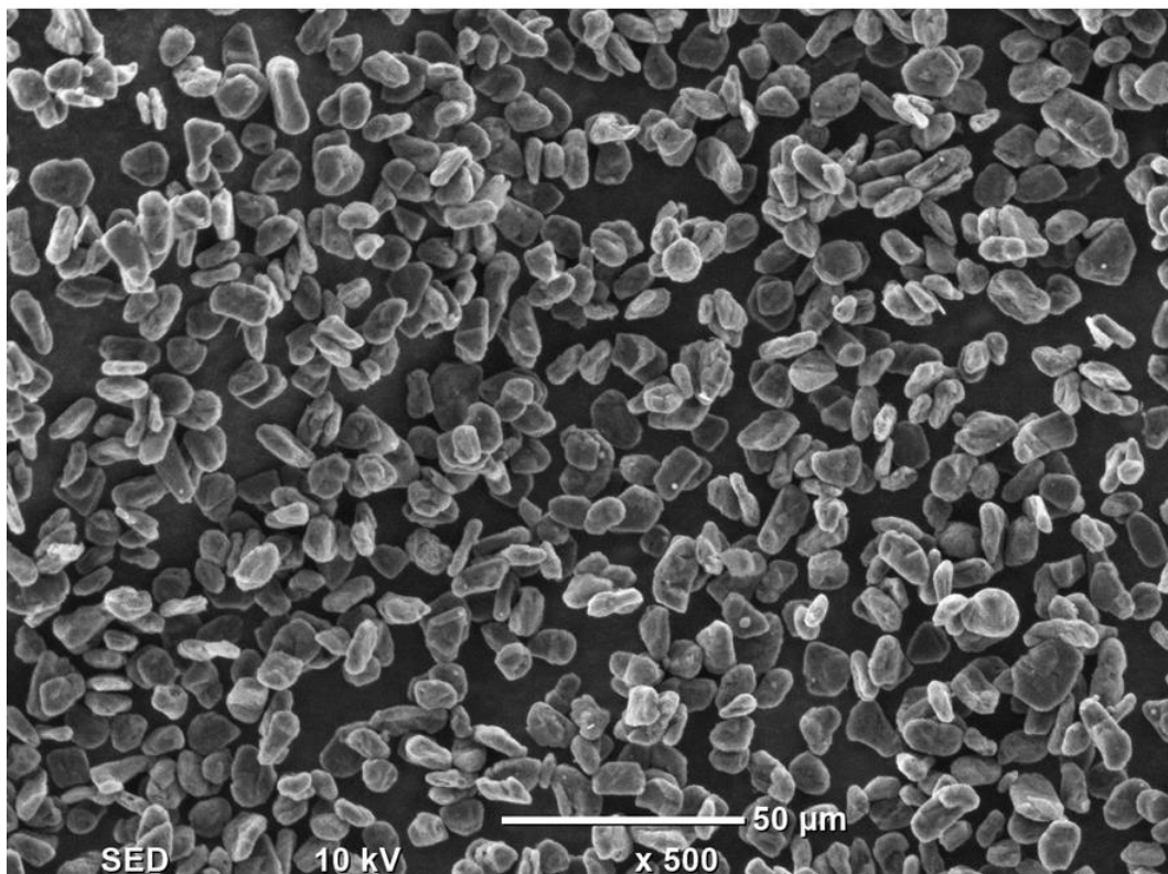
LT-N2 天然石墨电镜图(SEM)
