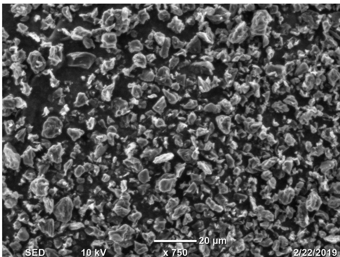
LT-AC 人造石墨电镜图(SEM)
