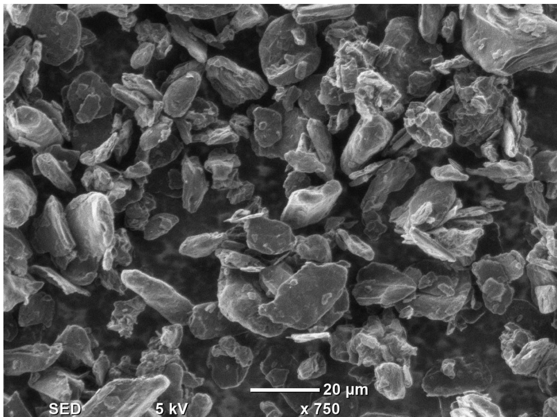
LT-A128HY 人造石墨电镜图(SEM)
