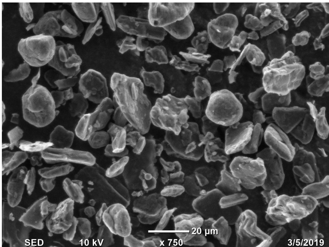
LT-A110P3 人造石墨电镜图(SEM)
