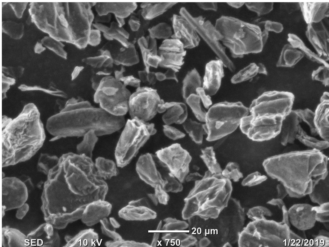
LT-A110K7 人造石墨电镜图(SEM)
