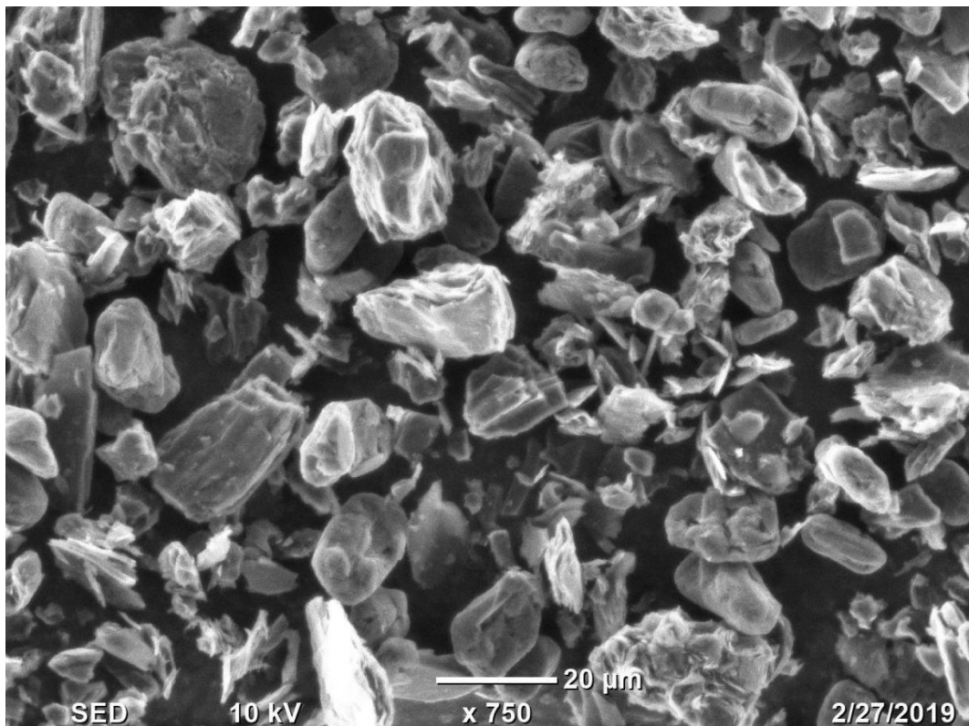
LT-A109-6 複合石墨电镜图(SEM)
