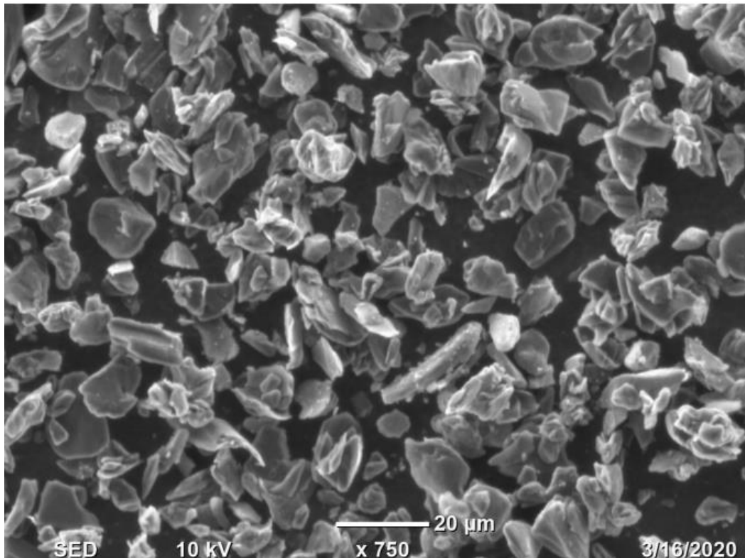
LT-ZH-9X-420 SiO/C (SEM)
